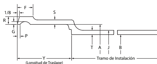
Tubería para Sistema Campana y Espiga de Hierro Fundido
